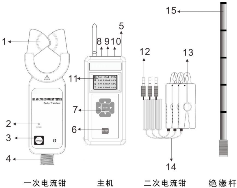
ETCR9500C-008 结构图
