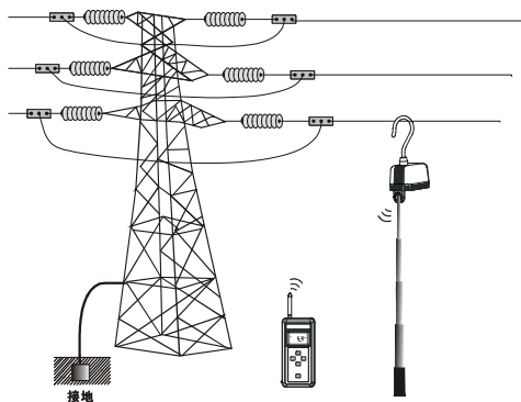
现场测试示意图
