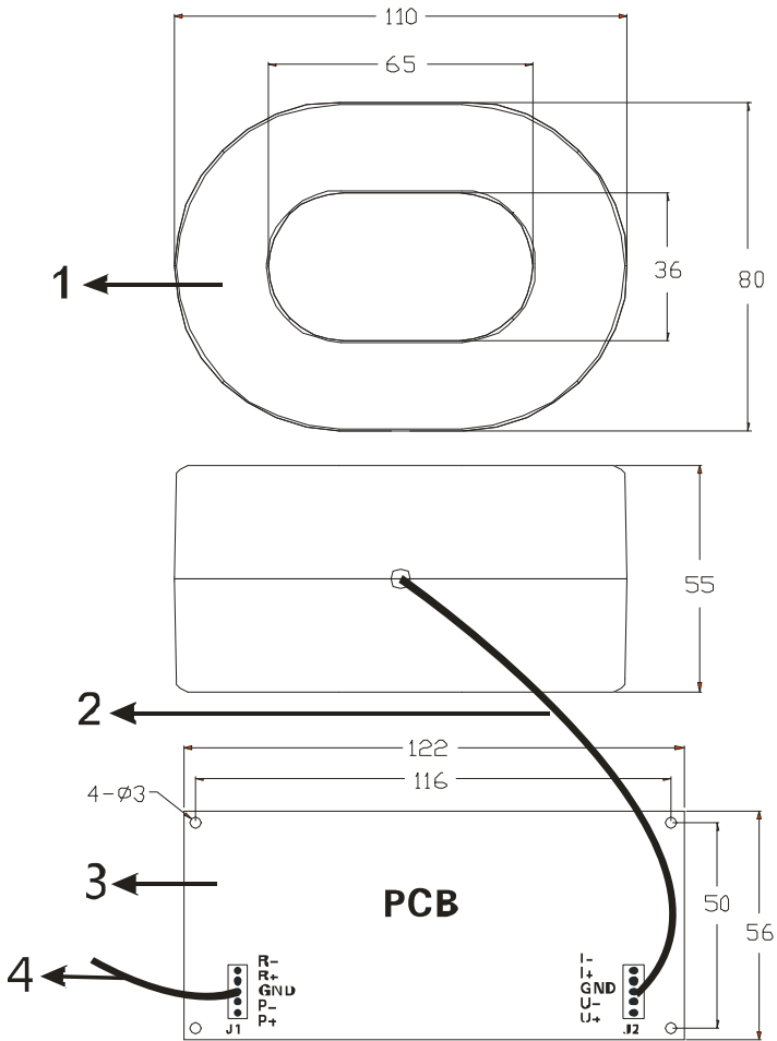
ETCR2800N 传感器结构尺寸
