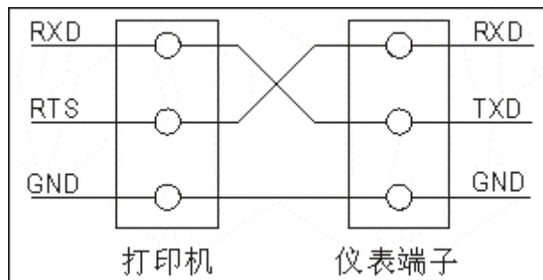
图 5.9 打印机接线图 8.2 操作
