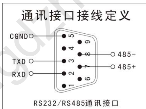
图6.4 通讯接线图
