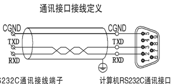
图 7.1 RS-232C 通讯接线方法
