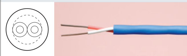
1 対丸型シリコンゴム被覆 0.65×1P K-2-SR-J2=KKT (0.65×1P K-SR=KKT)
