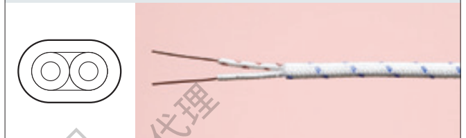
1 対平型セラミック編組被覆 0.32×1P K-CERAC
