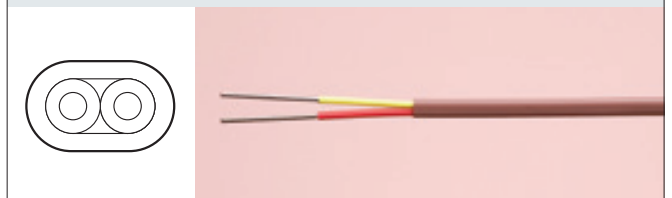
UL 規格認証 1 対平型 PFA 被覆 AWG23 (0.65mm) × 1P K-ASt-PFA-AS-[RU]
