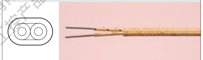
1 対平型シリカガラス編組被覆 0.65×1P K-SLGB
