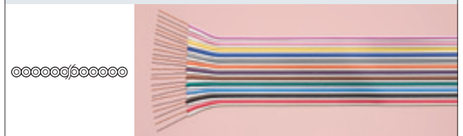
リボン型ビニル被覆 0.32×12P T-G = r
