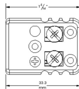
Jab-In 陶瓷插座 45C1XX00 XX= 分度号编号
