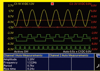
波形与逻辑电平
