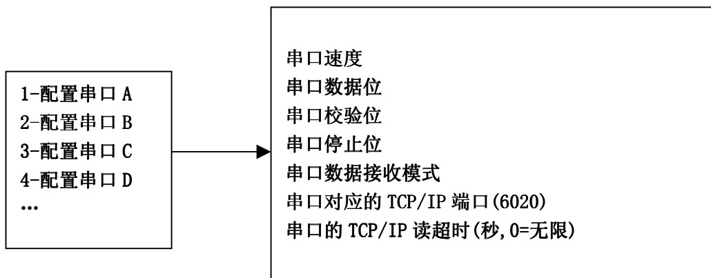
Server 模式串口服务器端口配置菜单结构
