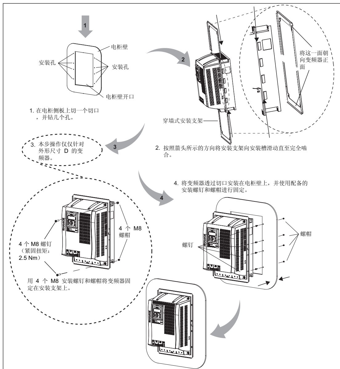
图 5-9 穿墙式安装变频器（举例）
