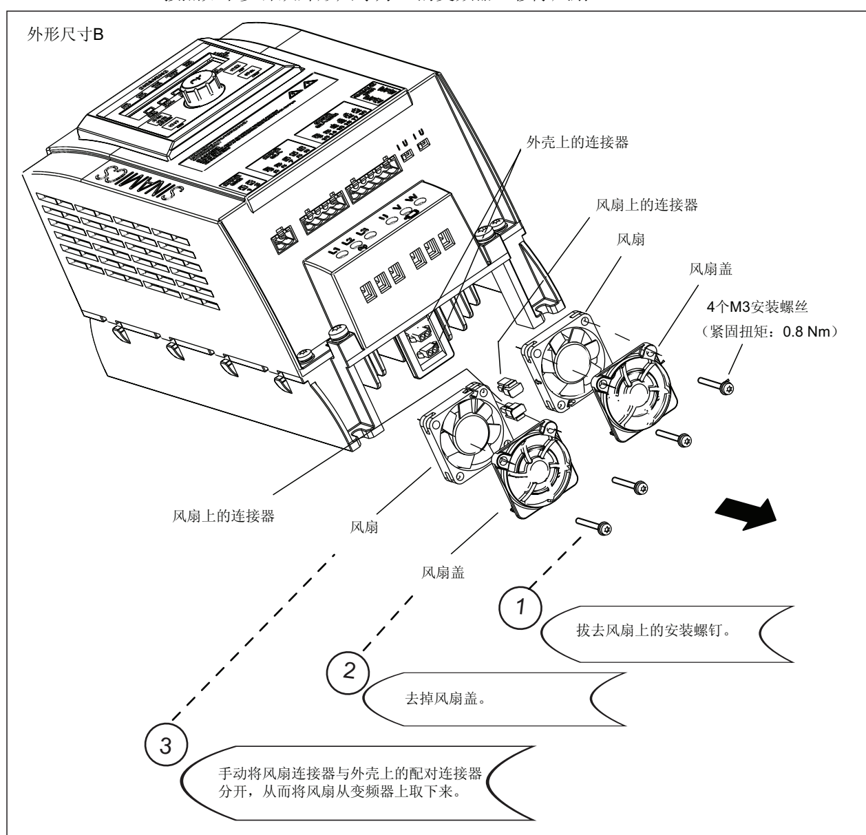
图 A-1 更换外形尺寸为 B 的变频器上的风扇
