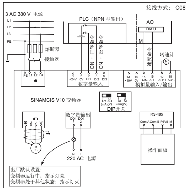
图 6-22 典型接线方式 8（C08）
