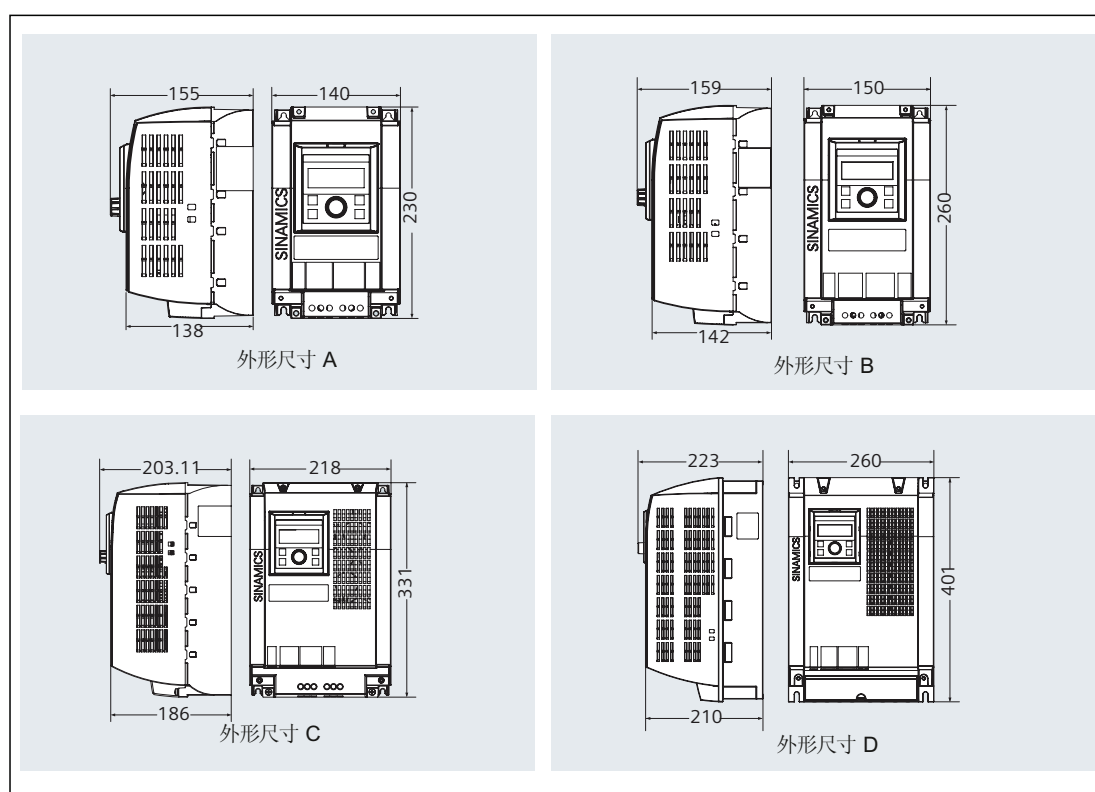
图 5-6 SINAMICS V10 的外形尺寸 (单位: mm)
