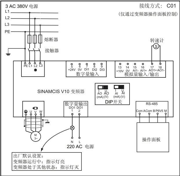
图 6-15 典型接线方式 1 (C01)
