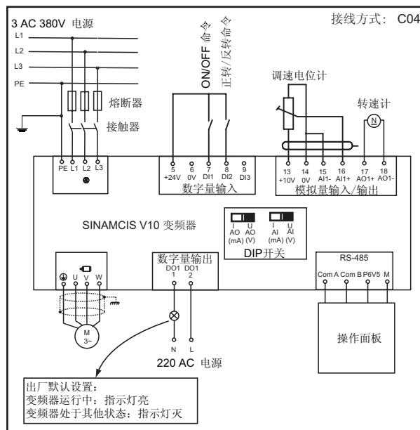
图 6-18 典型接线方式 4（C04）
