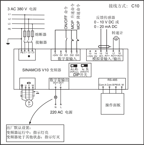
图 6-24 典型接线方式 10（C10）
