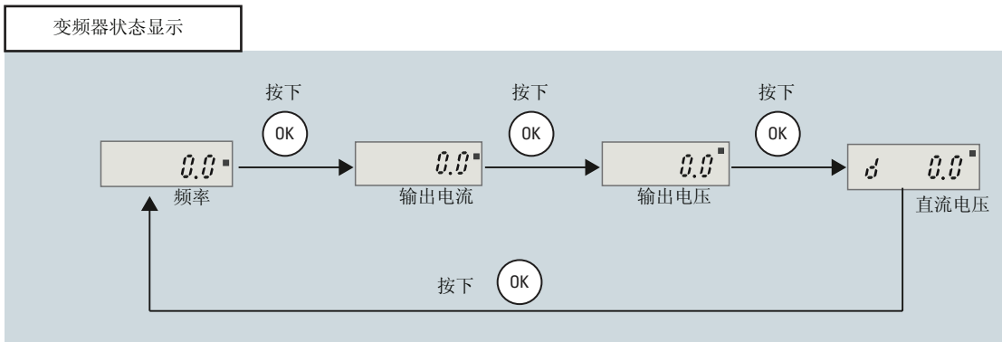
图 6-5 变频器的状态显示
