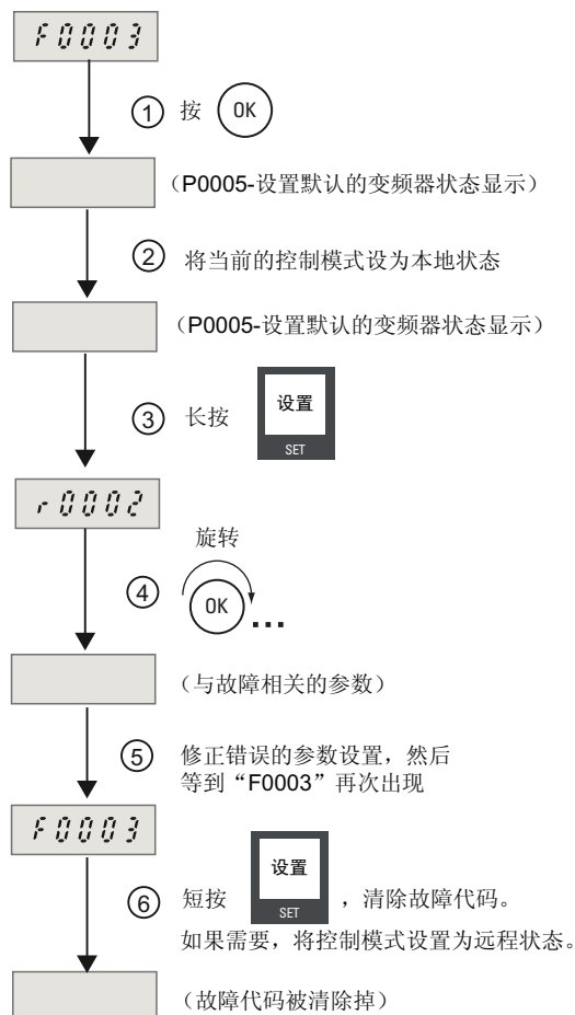
图 8-1 应答并清除 F0003（举例）
