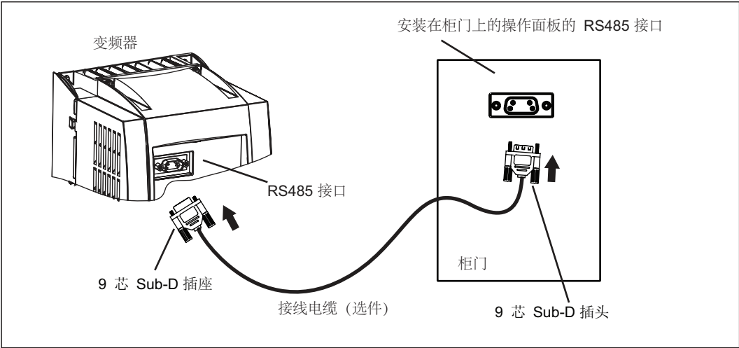
图 5-14 变频器主机和远程操作面板之间的接口
