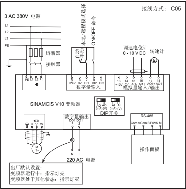
图 6-19 典型接线方式 5（C05）
