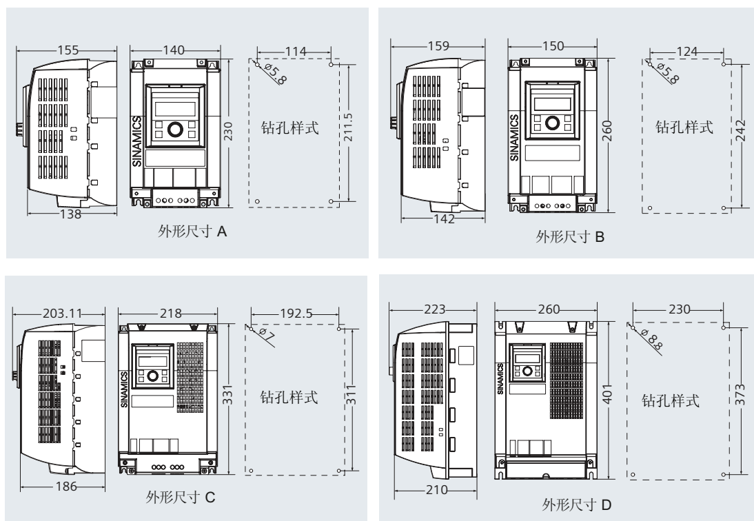
图 5-4 安装尺寸 (单位: mm)
