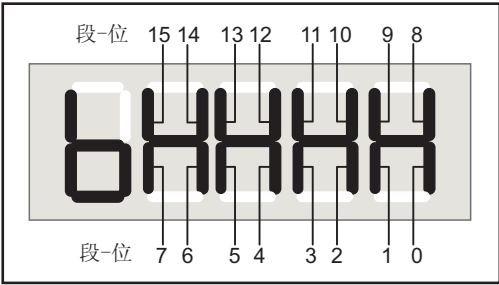
图 6-2 二进制参数显示
