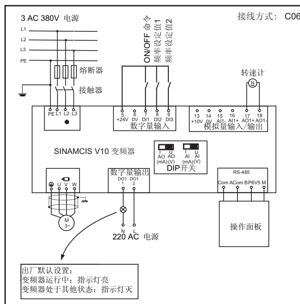
图 6-20 典型接线方式 6（C06）
