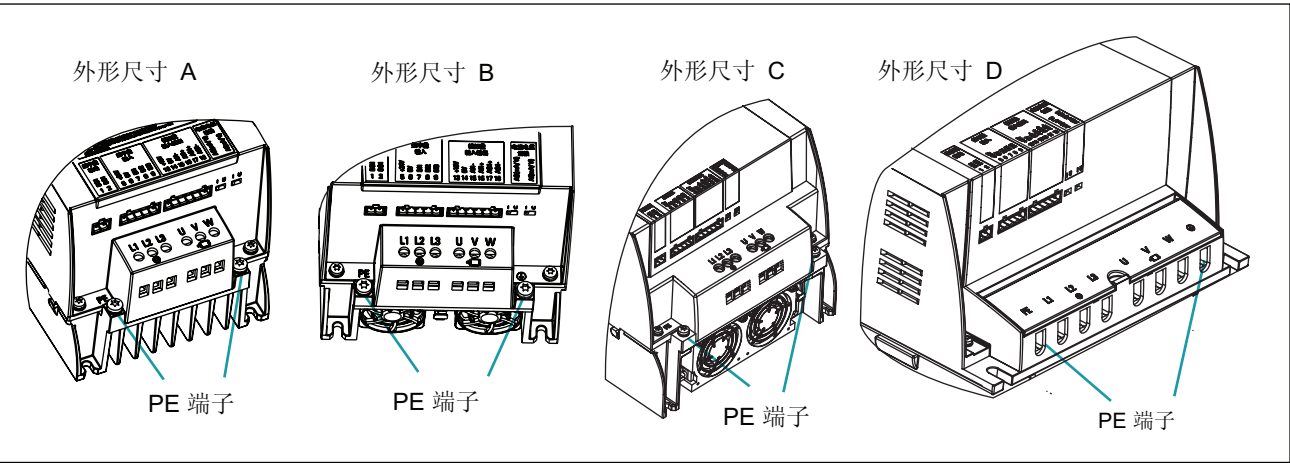
图 5-12 PE 端子布局
