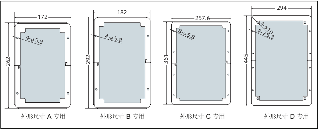
图 5-8 安装支架（选件）的外形尺寸（单位：mm）
