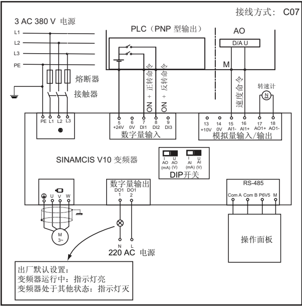
图 6-21 典型接线方式 7（C07）
