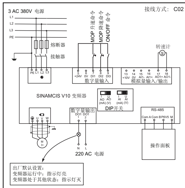
图 6-16 典型接线方式 2（C02）
