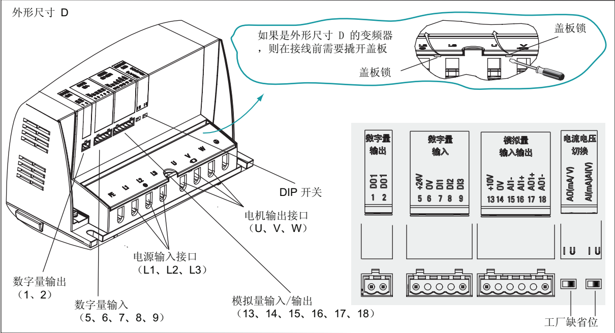
图 5-13 除 PE 端子之外的接口布局（举例）
