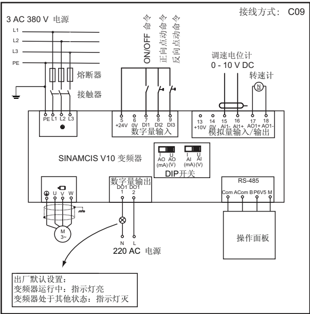
图 6-23 典型接线方式 9（C09）
