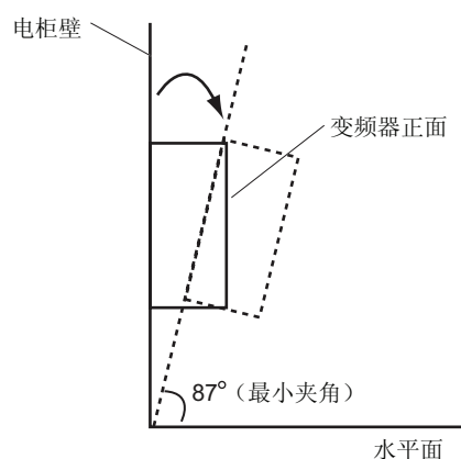
图 5-2 允许的安裝夾角
