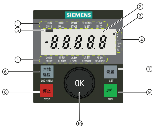
图 6-1 操作面板概览
