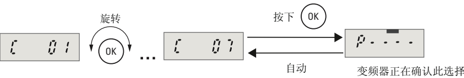
图 6-10 设置接线方式代码举例（C07）
