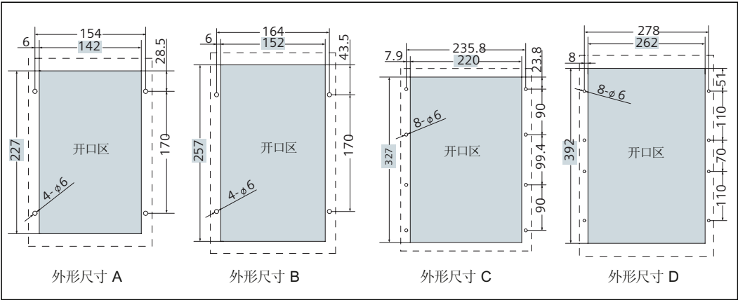
图 5-7 钻孔样式和开口尺寸（单位：mm）
