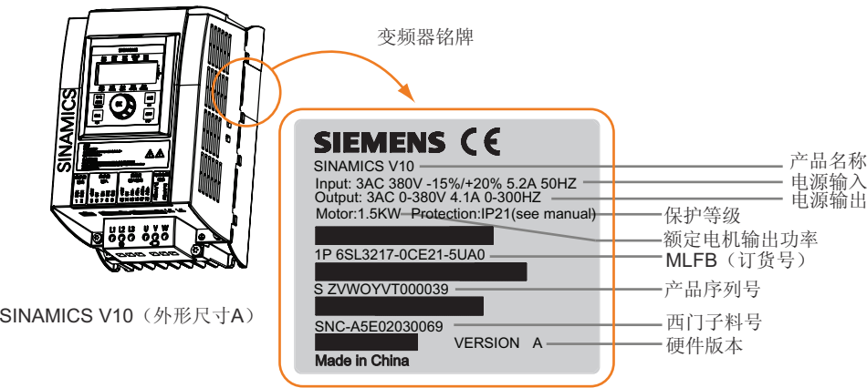
图 4-1 变频器铭牌（举例）
