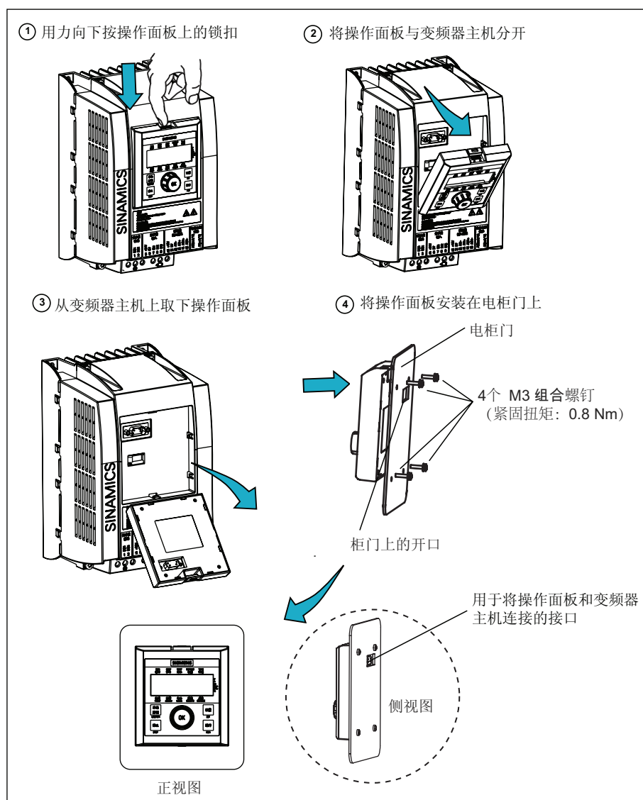
图 5-11 将操作面板安装在柜门上的步骤
