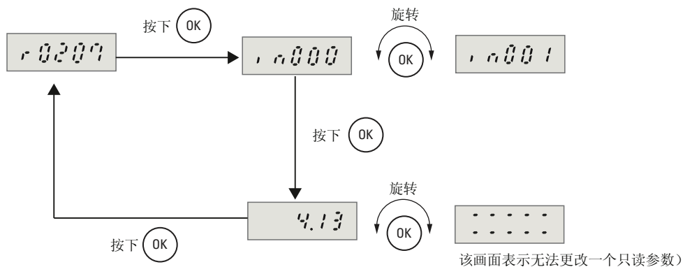
图 6-13 设置一个下标参数（举例）
