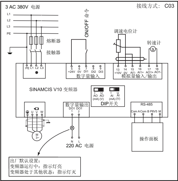
图 6-17 典型接线方式 3（C03）
