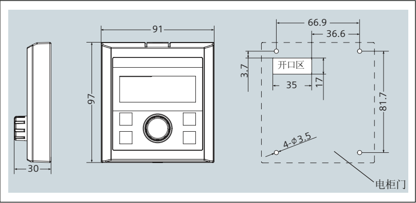
图 5-10 安装尺寸（外形尺寸 + 钻孔样式 + 开口尺寸）
