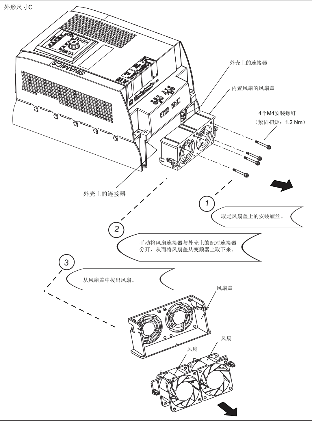
图 A-2 更换外形尺寸为 C 的变频器上的风扇
