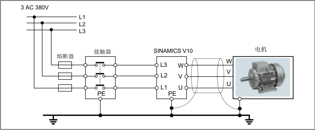
图 5-15 电源和电机的接线
