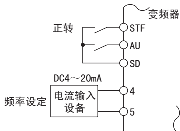
使用端子4(DC4~20mA)的接线图
