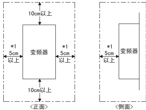
变频器周围的间隙
