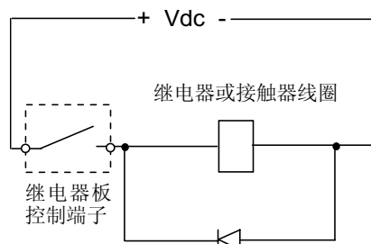
图3—7b 直流吸收电路
