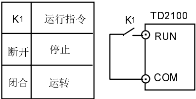
图6—21 普通控制模式
