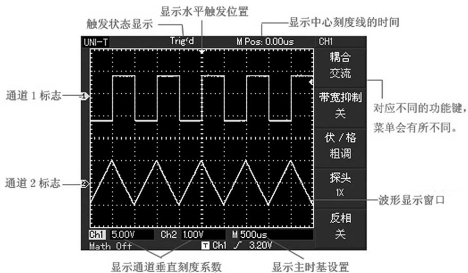
图1-3 显示界面说明图
