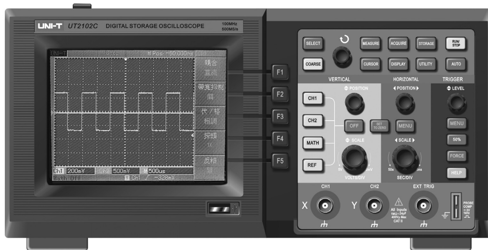
图1-1 UT2000/3000系列数字存储示波器前面板
