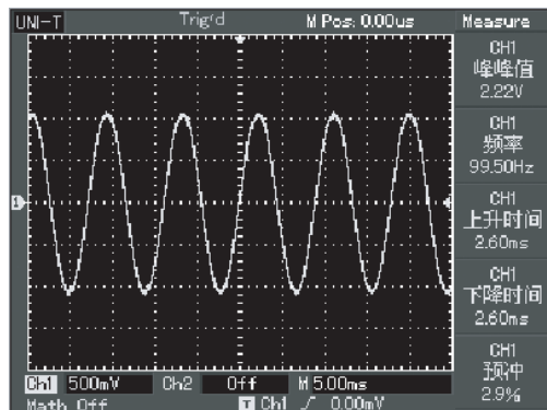
图3-1 自动测量
