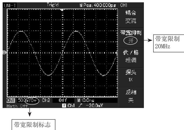
图2-5 带宽限制打开时的波形显示
