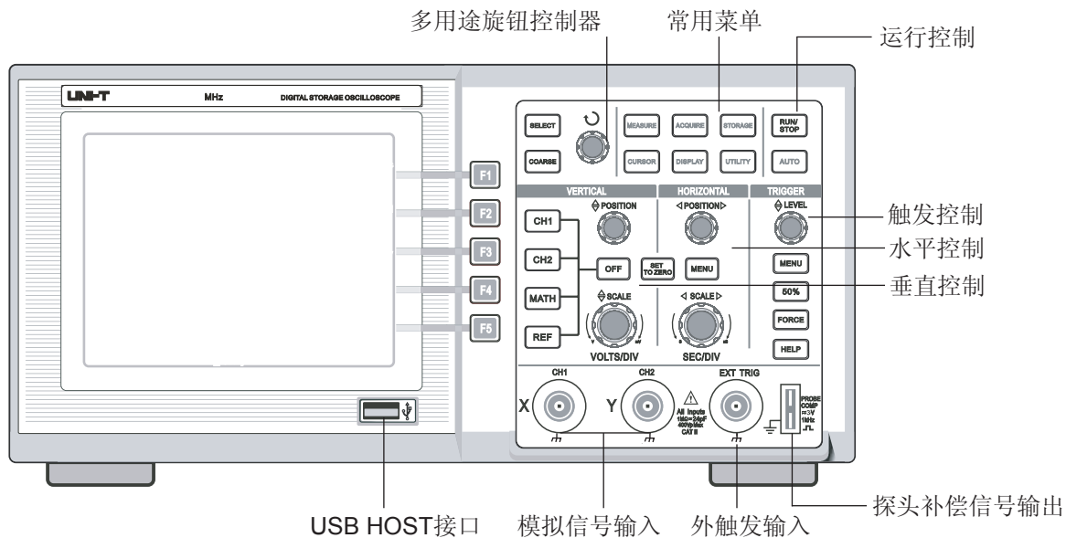
图1-2 UT2000/3000面板操作说明图
