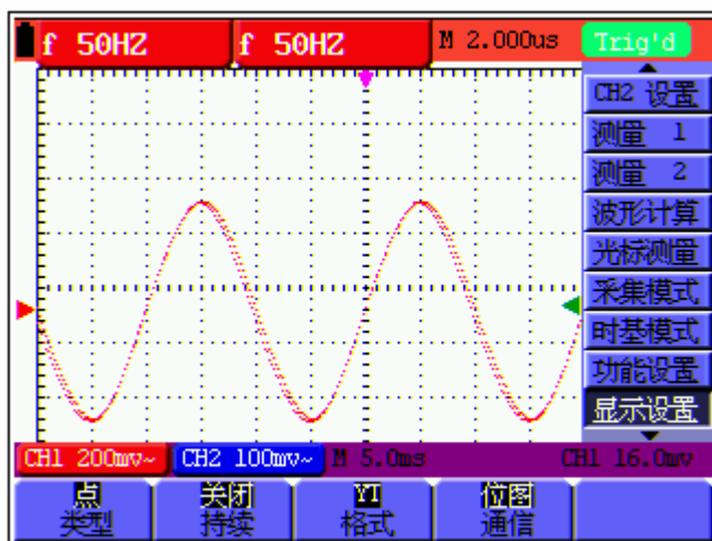
图 46：点显示
