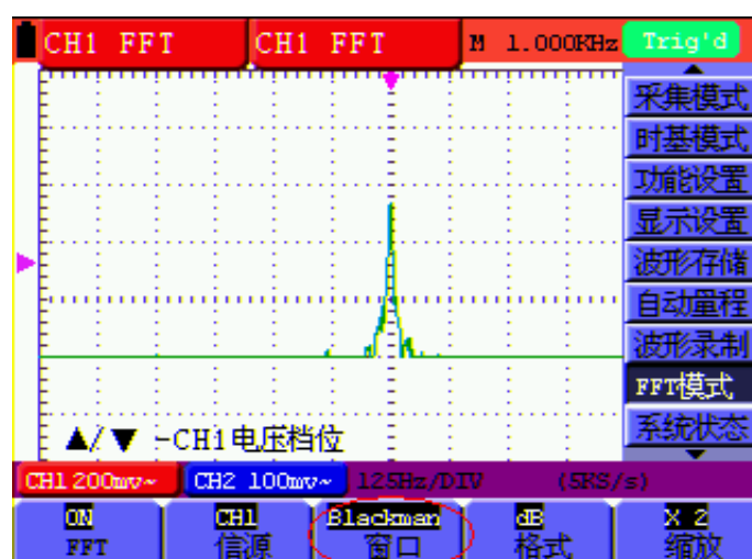
图61. BLACKMAN窗
