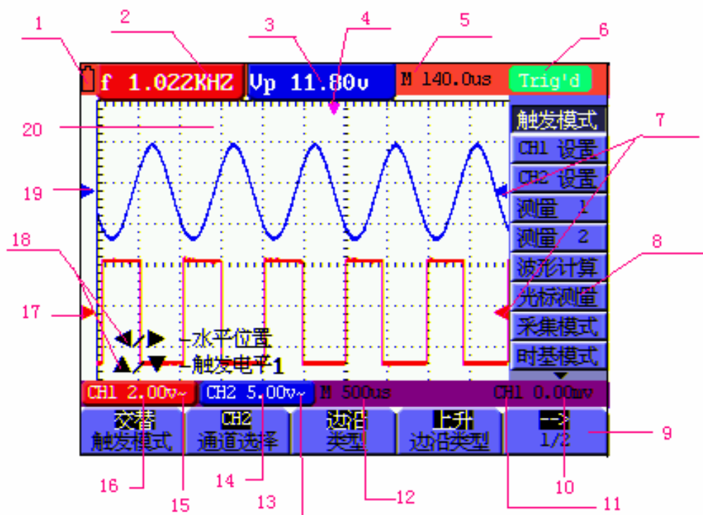
图 5：示波器界面
