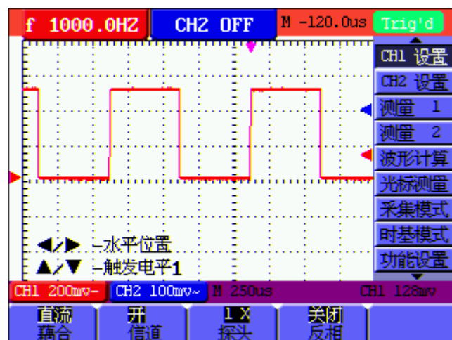
图 36: 直流耦合
