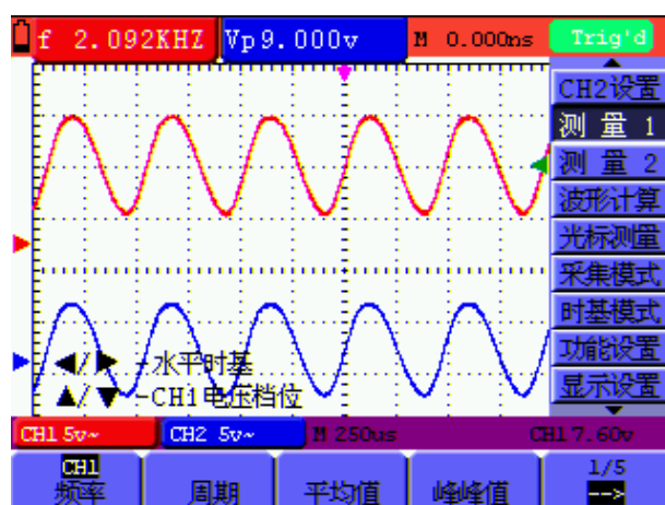
图 50: 自动测量
