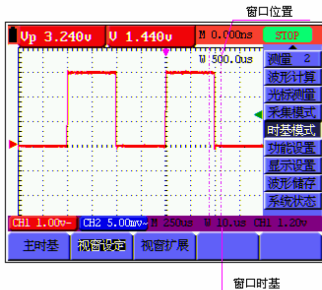
图58：视窗设定
