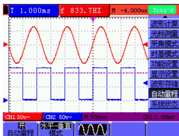
图 53 自动量程 水平---垂直模式多周期波形图
