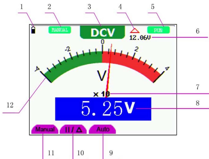
图 20：万用表界面
