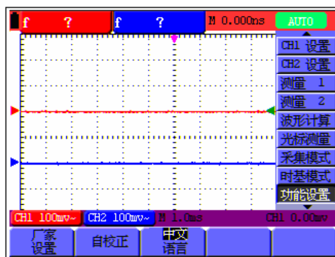
图 11：厂家设置
