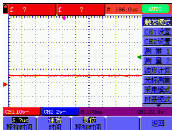
图46：触发释抑
