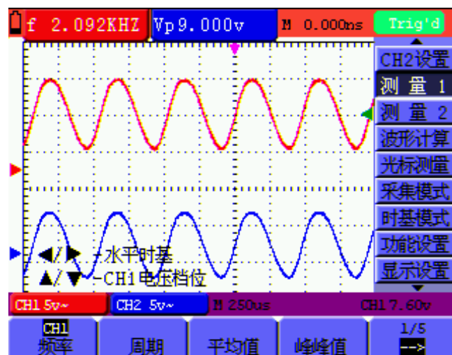
图 12：自动测量
