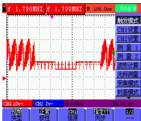
图44 视频指定行触发（第一页）
