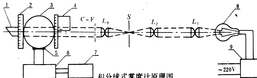
1—陷阱；2—标准板；3—积分球；4—试样架；5—光电池； 6—控制线路；7—检流计；8—光源；9—稳压器 L_1 、 L_2 、 L_3 —透镜；S—光孔；C-F—滤光器
