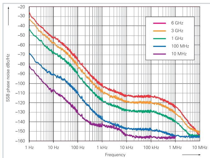
使用内部的OCXO（R&S®SMBV-B1 选项）测得的SSB相位噪声
