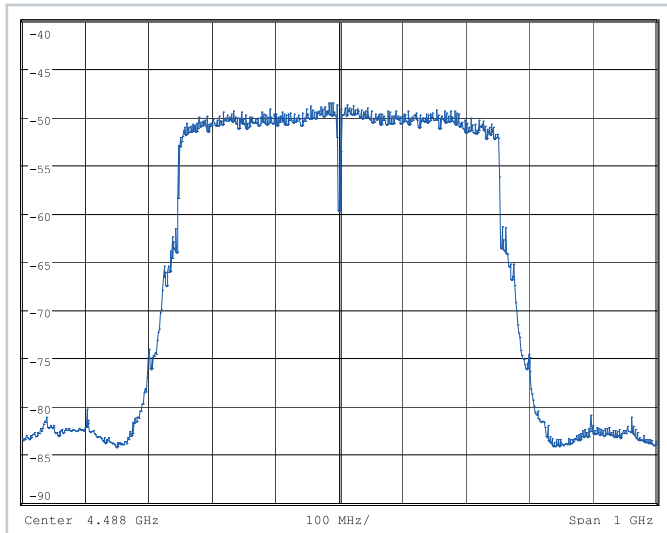
带宽超过500 MHz的I/Q调制器的频率响应
