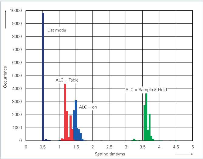
测得的 I/Q 模式下电平设置时间的柱状图
