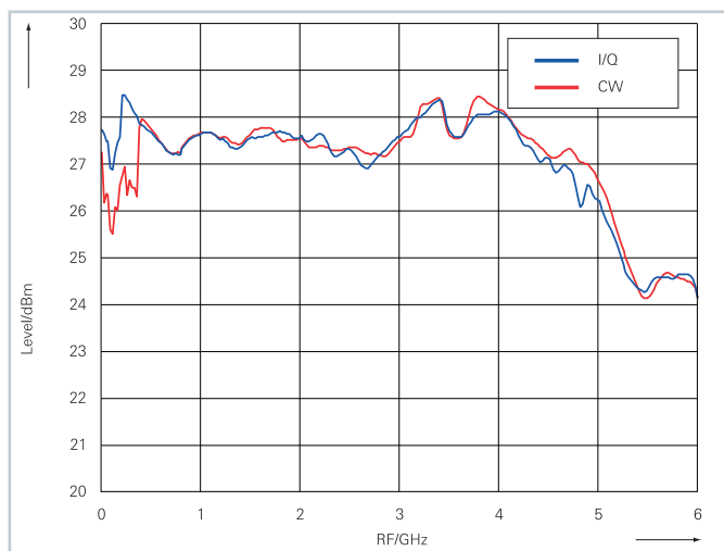
测得的最大输出功率/频率图
