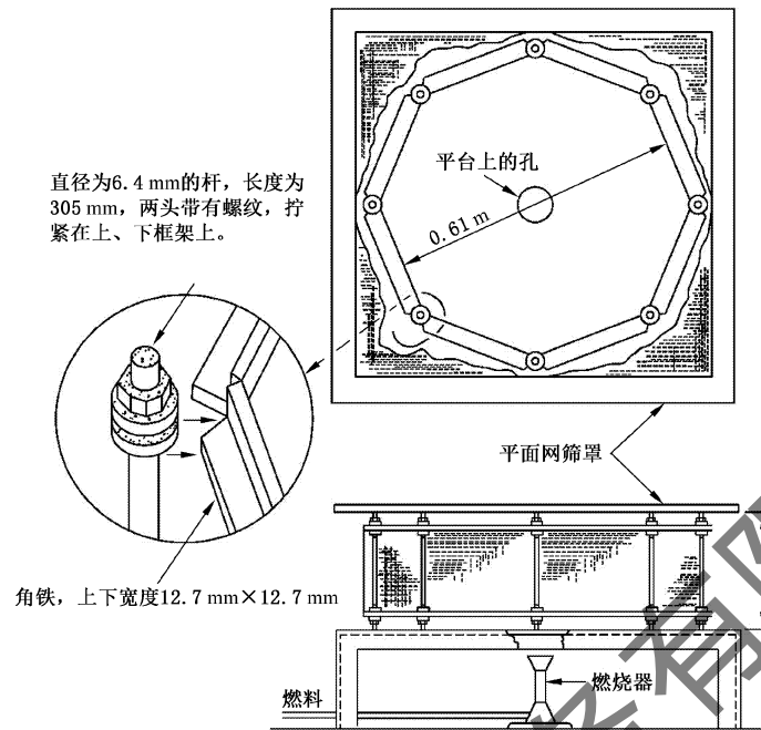
图 E.2 燃烧试验工装
