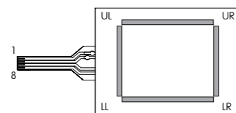
UL, LL, UR, LR: 下部电极端子 SENSE: 上部电极端子
