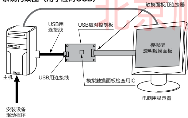
系统构成图 (用于应对USB)
