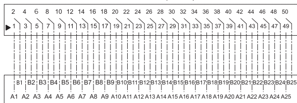
Terminal Block(端子部)
