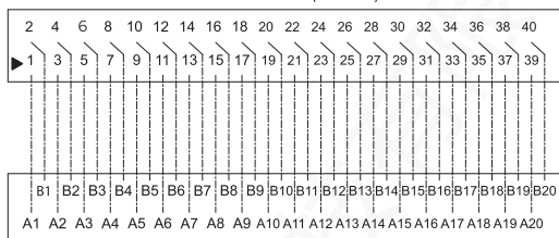
Terminal Block(端子部)
