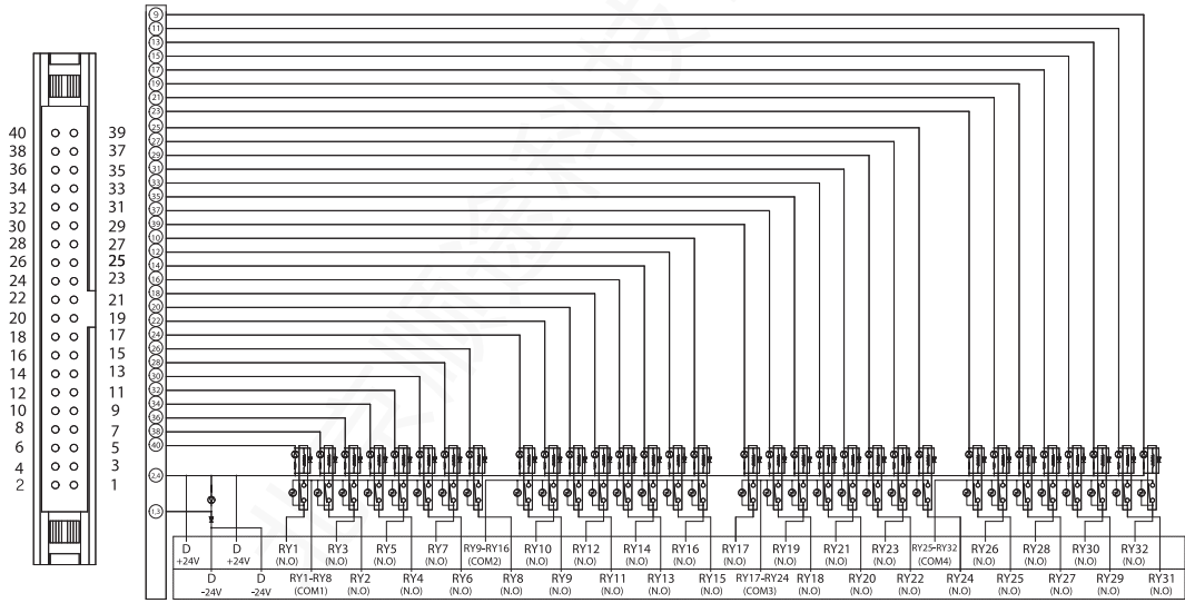
接线图
