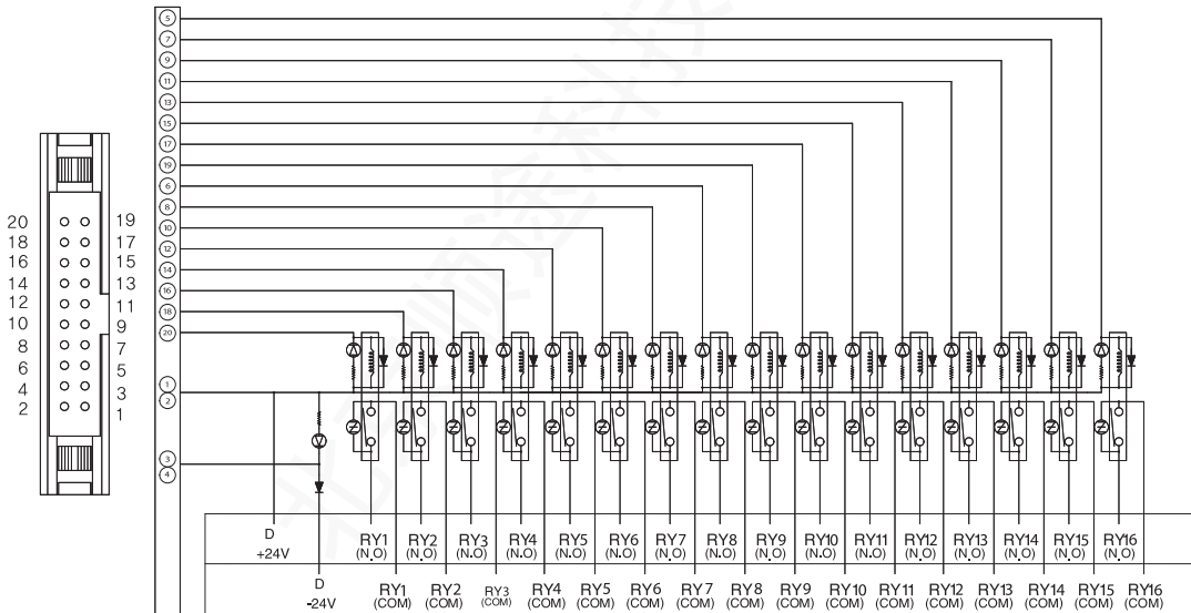
接线图
