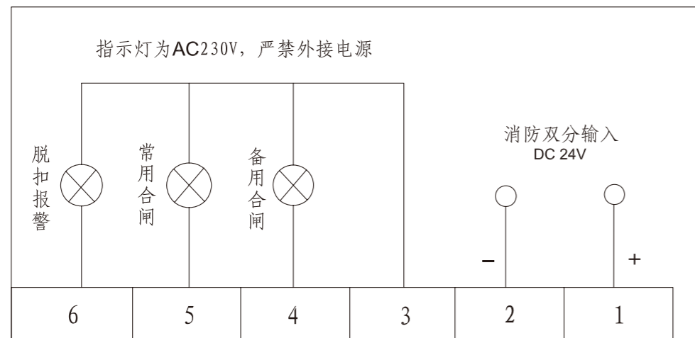
KWQ4-63二次接线端子图
