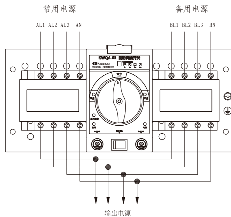
KWQ4-63主电路接线图
