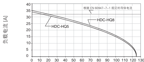
HDC-HQ5 和 HDC-HQ8 / H07V-K4.0 环境温度 [C]
