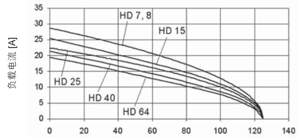
HD 车削式冷插针 2.5 mm 2 环境温度 [°C]
