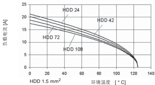
电流曲线
