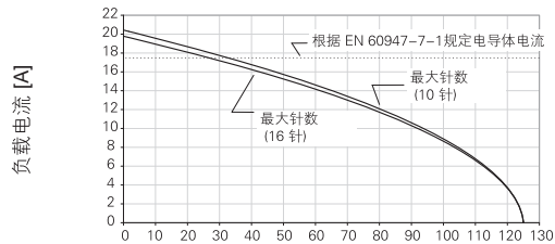
10 ... 48-针, 1.5 mm 2 环境温度 [°C]
