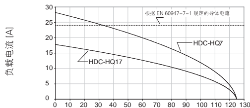
HDC-HQ7 and HDC-HQ17 / H07V-K2.5 环境温度 [C]
