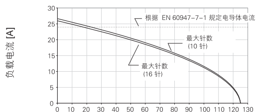
10 ... 48-针, 2.5 mm 2 环境温度 [°C]
