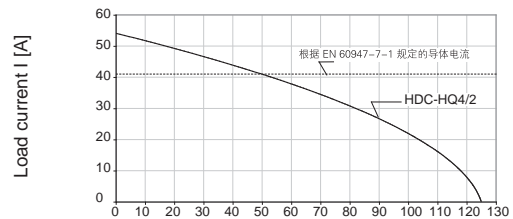
HDC-HQ4/2 / H07V-K6.0 环境温度 [C]
