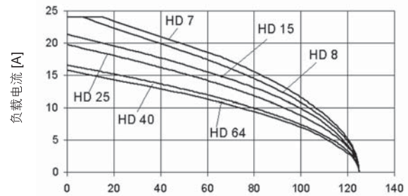
HD 车削式冷插针 1.5 mm 2 环境温度 [°C]
