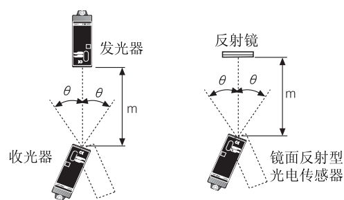
※m: 检测距离, \theta : 传感器角度
