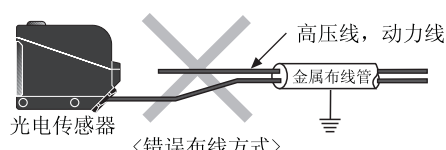
＜错误布线方式＞
