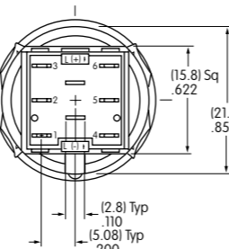
单极型号没有端子4, 5和6。
