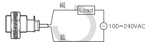
< 交流2线型 >
