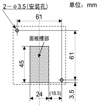
面板槽尺寸图 (A视图)
