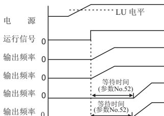
【电源接通后, 运行信号ON时】
