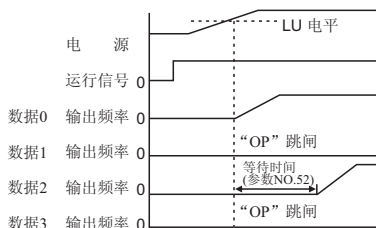
【运行信号接通状态下, 电源ON时】
