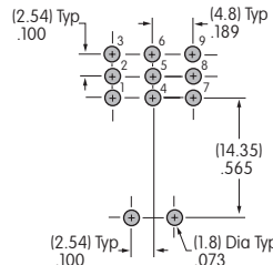
3极
