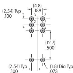
双极
