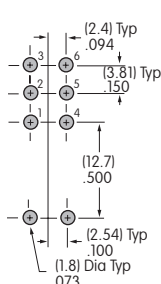
双极
