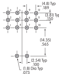
4极
