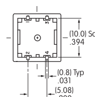
有框架的嵌入式盖帽 · 直型PC端子
