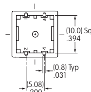
扁平嵌入式盖帽 · 直型PC端子
