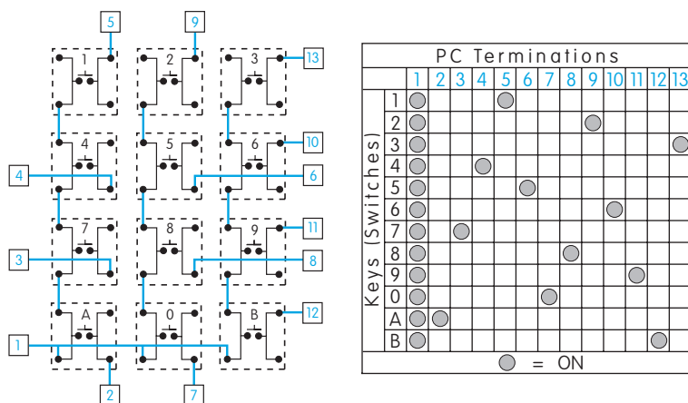
公共总线矩阵
