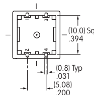
有刻纹的嵌入式盖帽 · 直型PC端子
