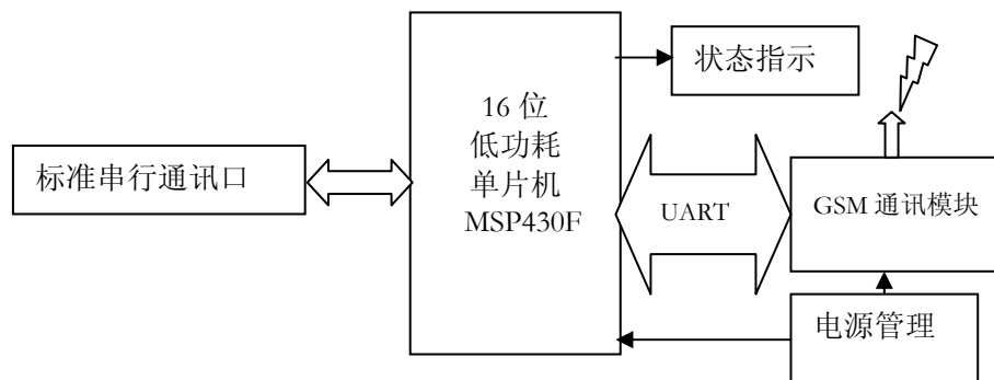
图 1. DTP-T05 系列 GSM 无线通信模块框图
