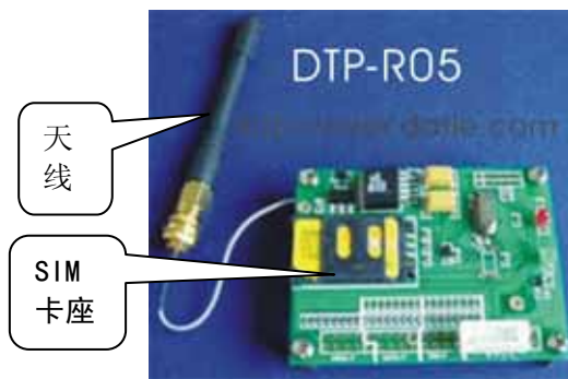
DTP-T05B 正面图
