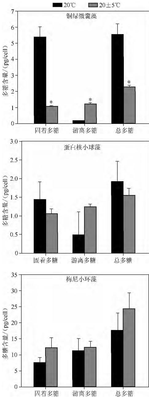
图3 铜绿微囊藻、蛋白核小球藻和梅尼小环藻在不同温度模式下固有多糖、游离多糖和总多糖的含量 (* 代表具有显著差异)
