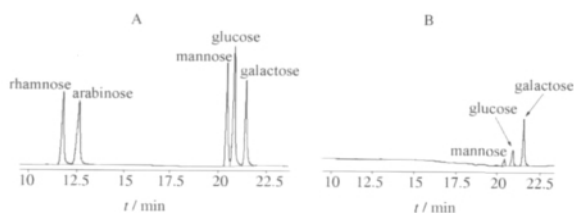
图 1 混合标准单糖(A)和 AOP1-1 水解产物(B)的气相色谱图 Fig. 1 Gas chromatograms of mixed standard monosaccharides (A) and hydrolyzed AP1-1 (B)
