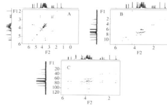
图 4 AP1-1 的 ^1\text{H} - ^1\text{H} COSY 谱(A), HSQC 谱(B)、HMBC 谱(C) Fig. 4 ^1\text{H} - ^1\text{H} COSY (A), HSQC (B) and HMBC (C) spectrum of AP1-1
