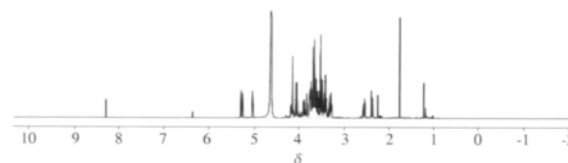
图 3 多糖 AP1-1 的 ^1\text{H} -NMR 谱 Fig. 3 ^1\text{H} -NMR Spectrum of AP1-1
