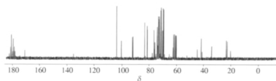
图 2 AP1-1 的 ^{13}\text{C} -NMR 谱 Fig. 2 ^{13}\text{C} -NMR Spectrum of AP1-1
