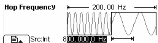
图 3- 10 输出FSK调制波形
