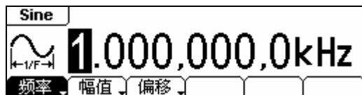
图 1- 10 正弦波常规显示界面
