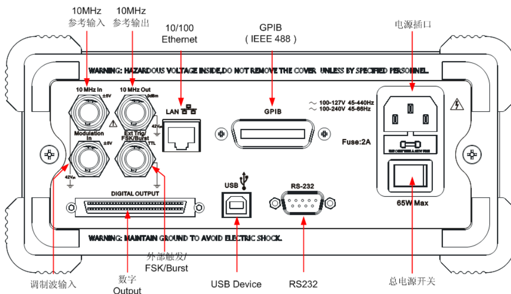
图 1-6 DG2000 系列函数/任意波形发生器后面板操作说明图
