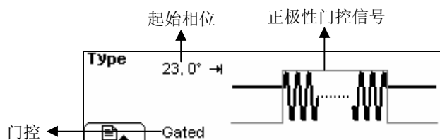
图 2- 62 图形显示模式下的波形参数
