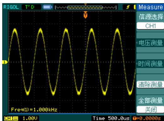
图 2- 69 DS1000中显示的波形
