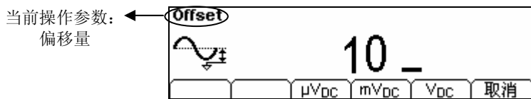
图 2- 7 设置偏移量的参数值
