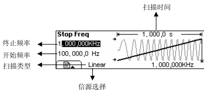
图 2- 57 图形显示模式下的波形参数
