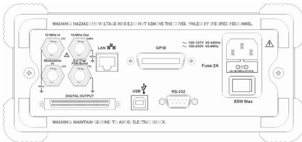
图 1-5 DG2000 系列函数/任意波形发生器后面板
