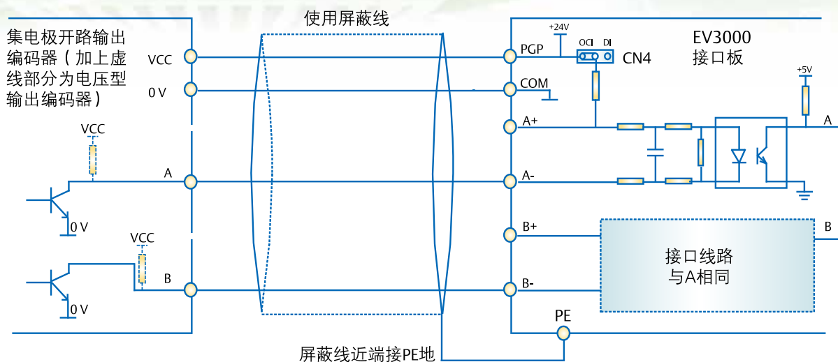
集电极开路输出编码器(加上虚线为电压型输出编码器)接线图
