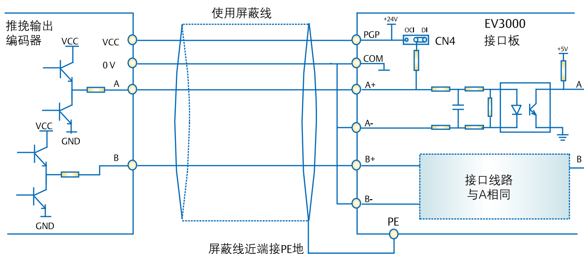
推挽输出编码器接线图
