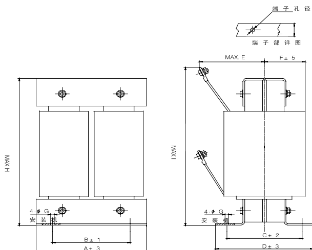
直流电抗器的外形图
