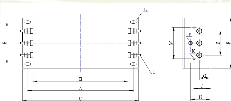
附图 5 EMI 滤波器外形图
