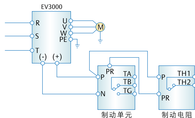
变频器与制动组件连接图
