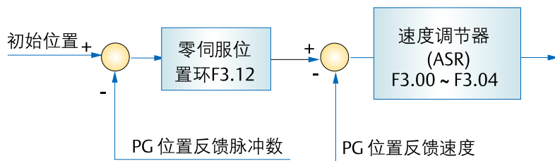
零伺服功能简化框图
