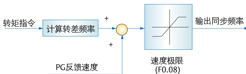
转矩控制功能框图
