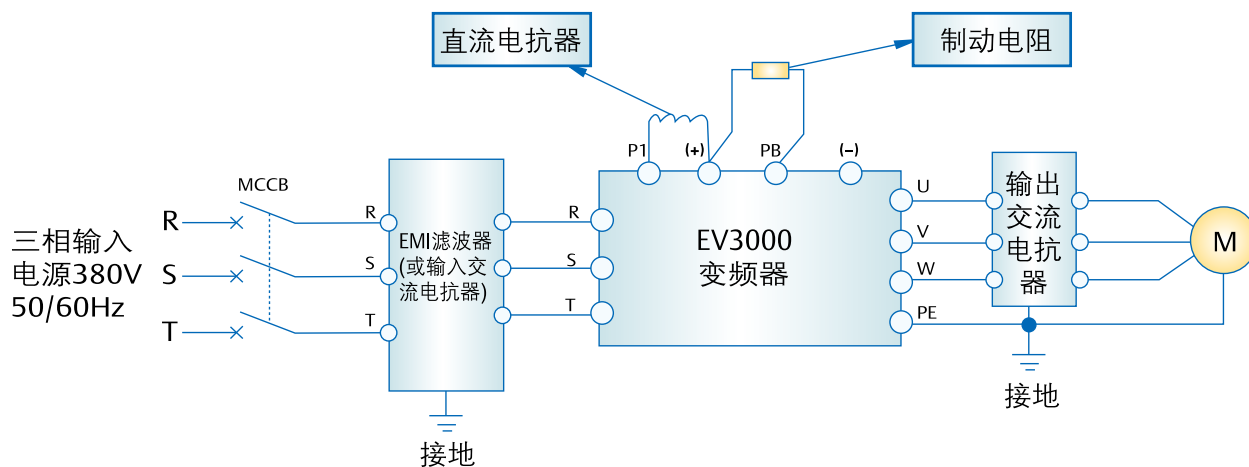
EV3000 变频器选配件接线示意图
