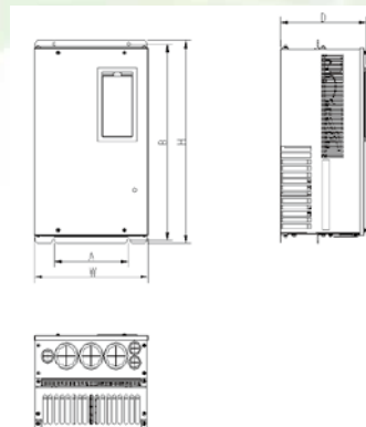
图 b EV3000-4T0185G ~ EV3000-4T0220G
