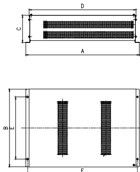
制动单元的安装尺寸示意图 制动电阻的安装尺寸示意图
