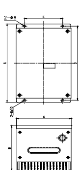
制动单元的安装尺寸示意图 制动电阻的安装尺寸示意图
