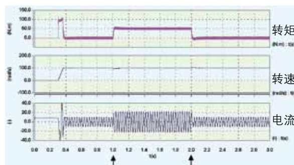
突加负载 突减负载 阶跃转矩响应特性(100%转矩)
