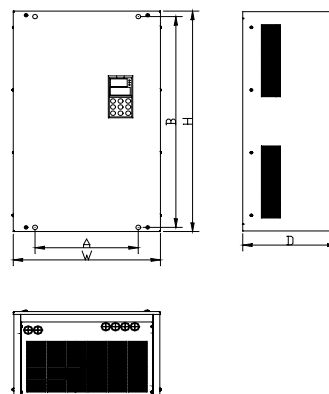
图 d EV3000-4T0550G ~ EV3000-4T0900G
