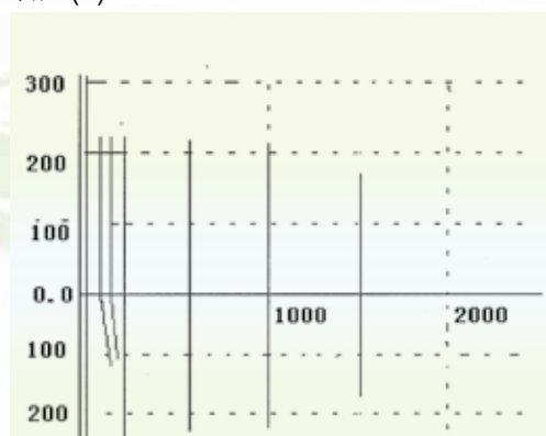
转矩 - 转速特性
