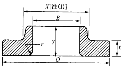
活套法兰
