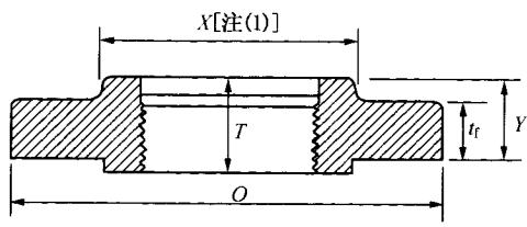
螺纹式法兰
