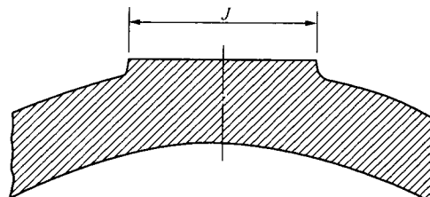
图 F5 连接件对接焊
