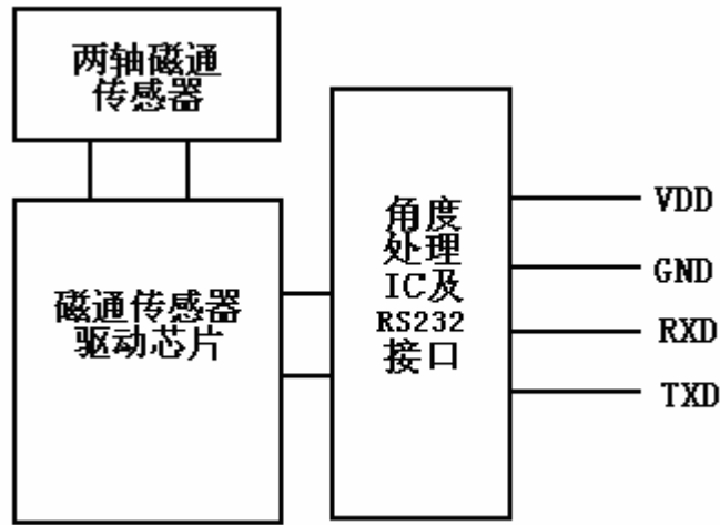
图(1) FAD-DCM-RS232 电路框图
