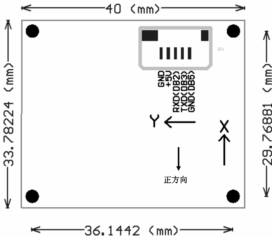
图(2) FAD-DCM-RS232 接线图
